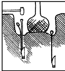
plaatsen van de grondankers
