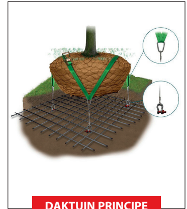
DAKTUIN PRINCIPE
